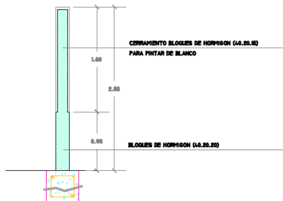
SECCION
